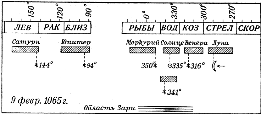
Рис. 150. Второе, окончательное, решение (Н. А. Морозова). Удовлетворительны все положения планет, где звездочки (планеты) находятся под своей полоской. В нижнем гороскопе, как единственно наблюдавшемся автором, все безусловно верно. А в верхнем вычисленном в 1065 году для 1049 (т. е. за 16 лет назад) Марс и Венера попали левее надлежащих мест вследствие неточного знания автором их синодического обращения.
