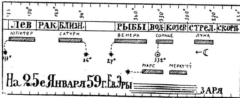
Рис. 147. Вильевский вариант вычислений Клобе'я (считая птицу со змеиным хвостом за Юпитера и птицу с бычьей головой за Сатурна). Удовлетворительны только те положения планет, где звездочка находится над своей полоской. Здесь в верхней полосе неудовлетворительны Юпитер, Марс и Солнце; в средней Венера и Меркурий; в нижней плохи Сатурн и Венера и неудовлетворителен Марс. Координаты 1910 года находятся под затушеванными полосками.
