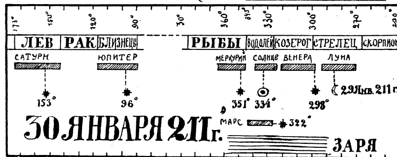
Рис. 149. Наглядное изображение результатов определения времени Атрибских гороскопов при предположении, что птица со змеиным хвостом — Сатурн, а птица с бычьей головой — Юпитер. Плохо подходят Меркурий в верхнем и Марс в нижнем гороскопе.
