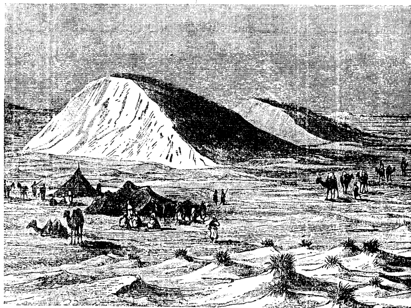
Рис. 129. Песчаные дюны в Сэхаре.
