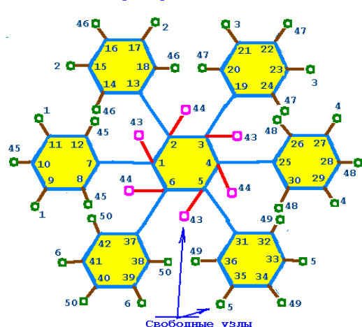
Бензольная структура золота
