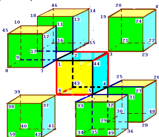
Кубическая решётка золота
